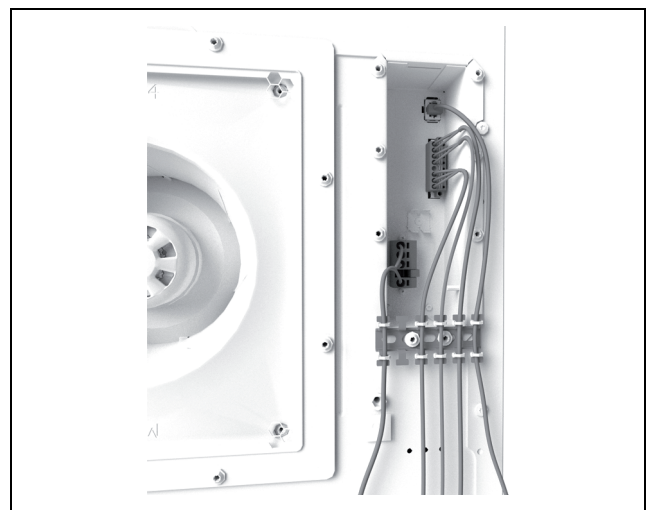
Fig. 40: Sistema di scarico della trazione con fascette serracavi (figura a titolo d'esempio)
