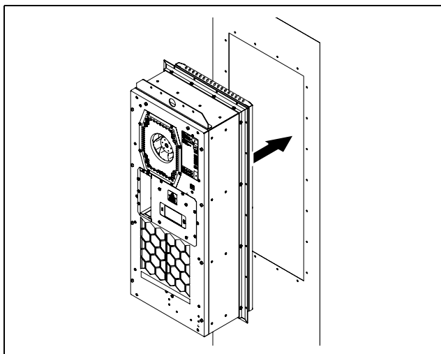
Fig. 25: Inserimento del condizionatore in una parte piana a parete singola
