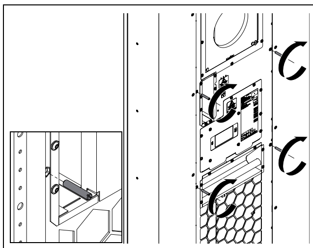
Bild 17: Skruva i gängbultarna i mitten
