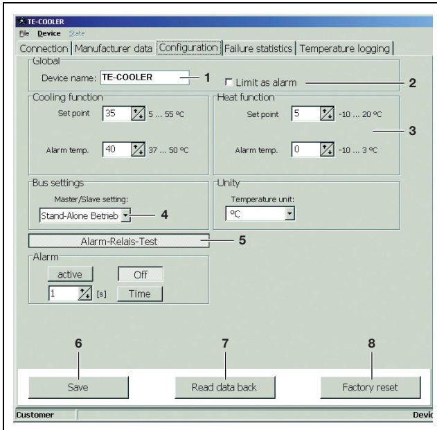
Obr. 22: Konfigurace RTC
