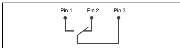
Obr. 24: Obsazení přepínacího kontaktu (ve stavu bez napětí)
