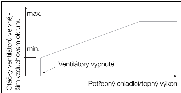
Obr. 3: Regulační chování ventilátorů ve vnějším vzduchovém okruhu
