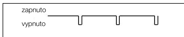
Obr. 24: Obsazení přepínacího kontaktu (ve stavu bez napětí)
