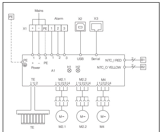
Obr. 13: Schéma elektrického zapojení č. 2, bez integrovaného síťového zdroje
