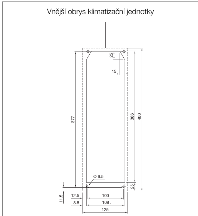
Obr. 28: Montážní výřez a rozměry otvorů při vnější montáži zařízení
