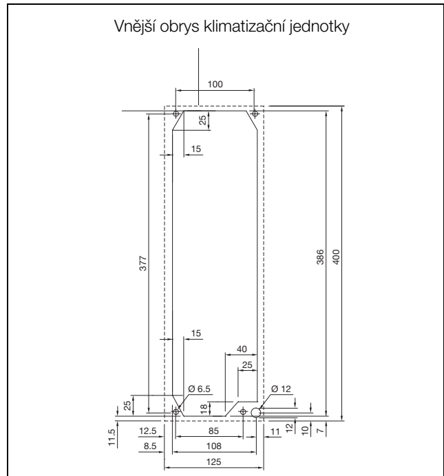
Obr. 29: Montážní výřez a rozměry otvorů při vestavbě zařízení (vnitřní montáž)
