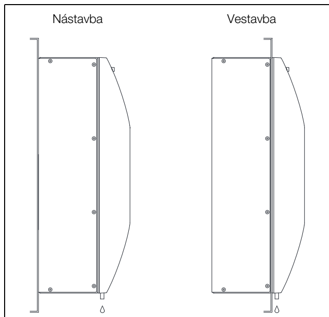
Obr. 4: Montáž zařízení jako nástavba a vestavba
