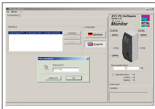
Obr. 21: Okno přihlášení
