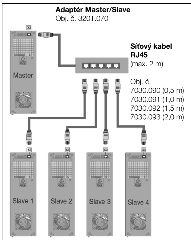
Obr. 11: Příklad připojení: provoz Master/Slave
