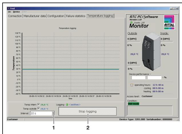
Obr. 25: Spuštění/ukončení záznamu teploty
