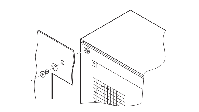
Obr. 6: Upevnění chladicí jednotky
