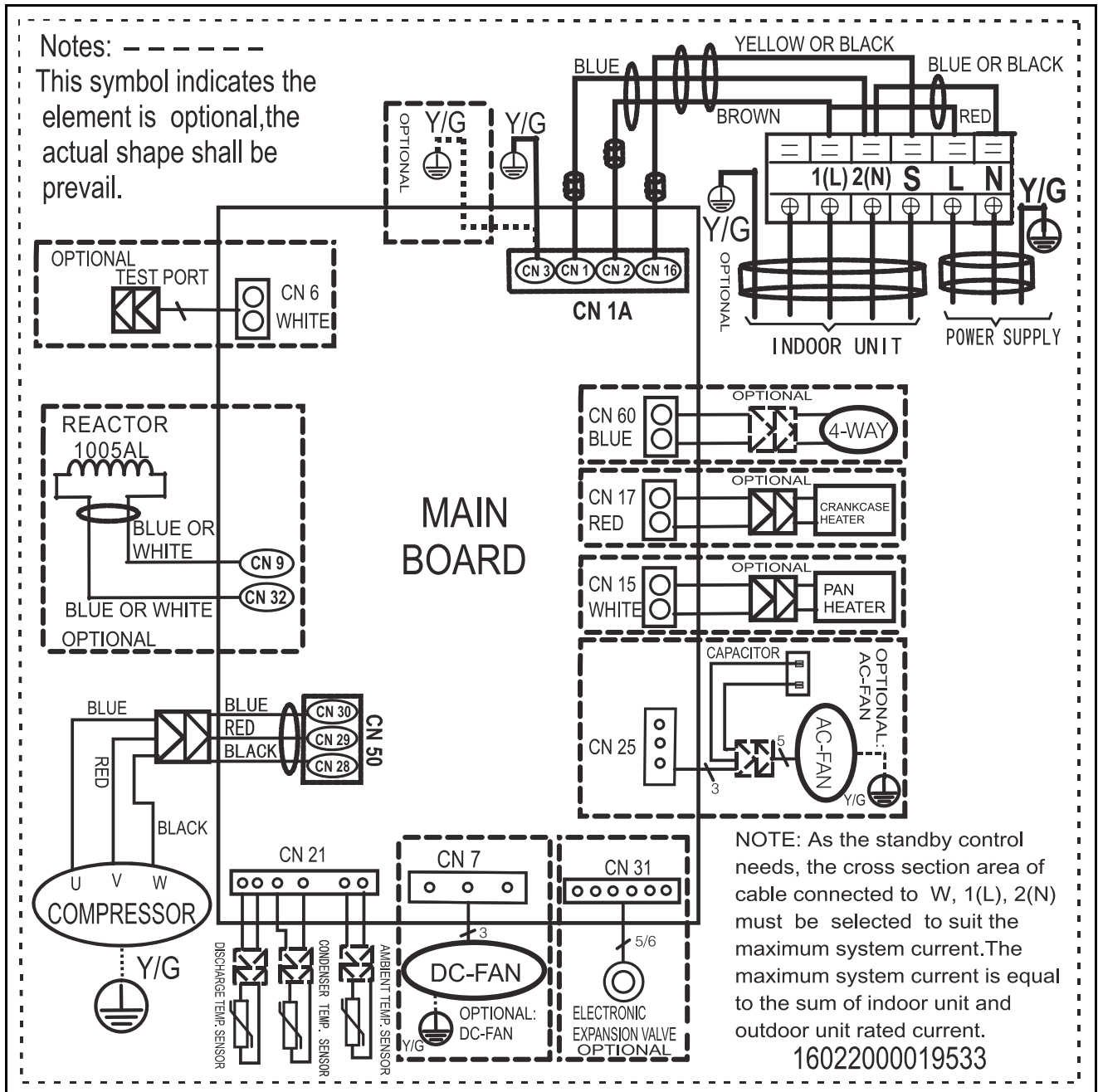
Abb. 27: Stromlaufplan Außeneinheit für 3 kW-Geräte (3311.490 und 3311.491)
