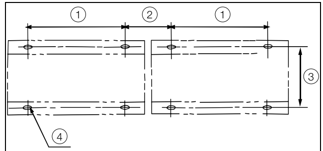
Abb. 9: Draufsicht Befestigungspunkte
