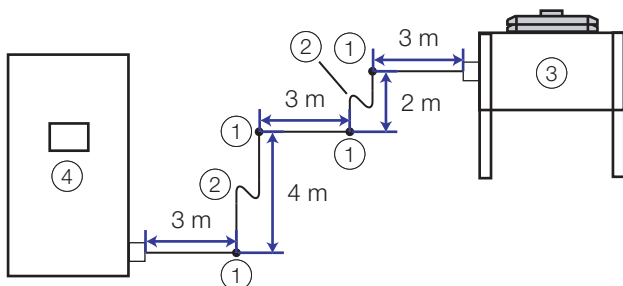
Abb. 19: Vereinfachte Darstellung der Anschlussleitungen
