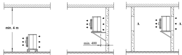
Abb. 15: Aufstellmöglichkeiten bei horizontalem Luftauslass
