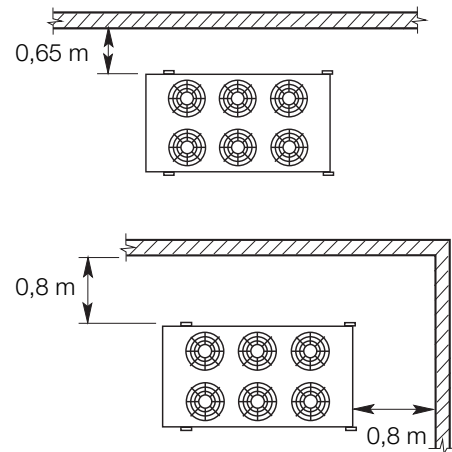
Abb. 14: Minimale Abstände bei vertikaler Montage
