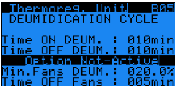
Abb. 62: Menü „B05“
