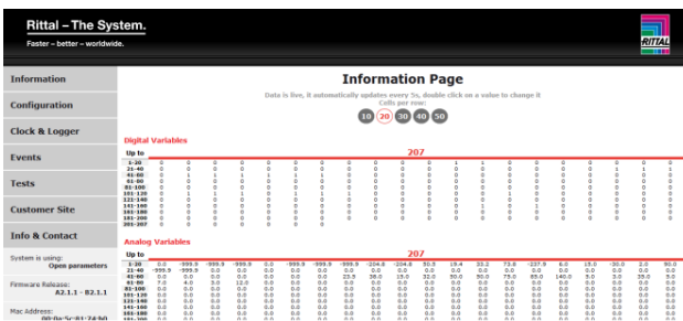
Abb. 52: Carel-Informationsseite
