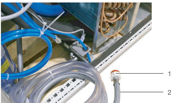
Abb. 55: Anschlusschlauch mit Anschlussstück 3/4" Außengewinde
