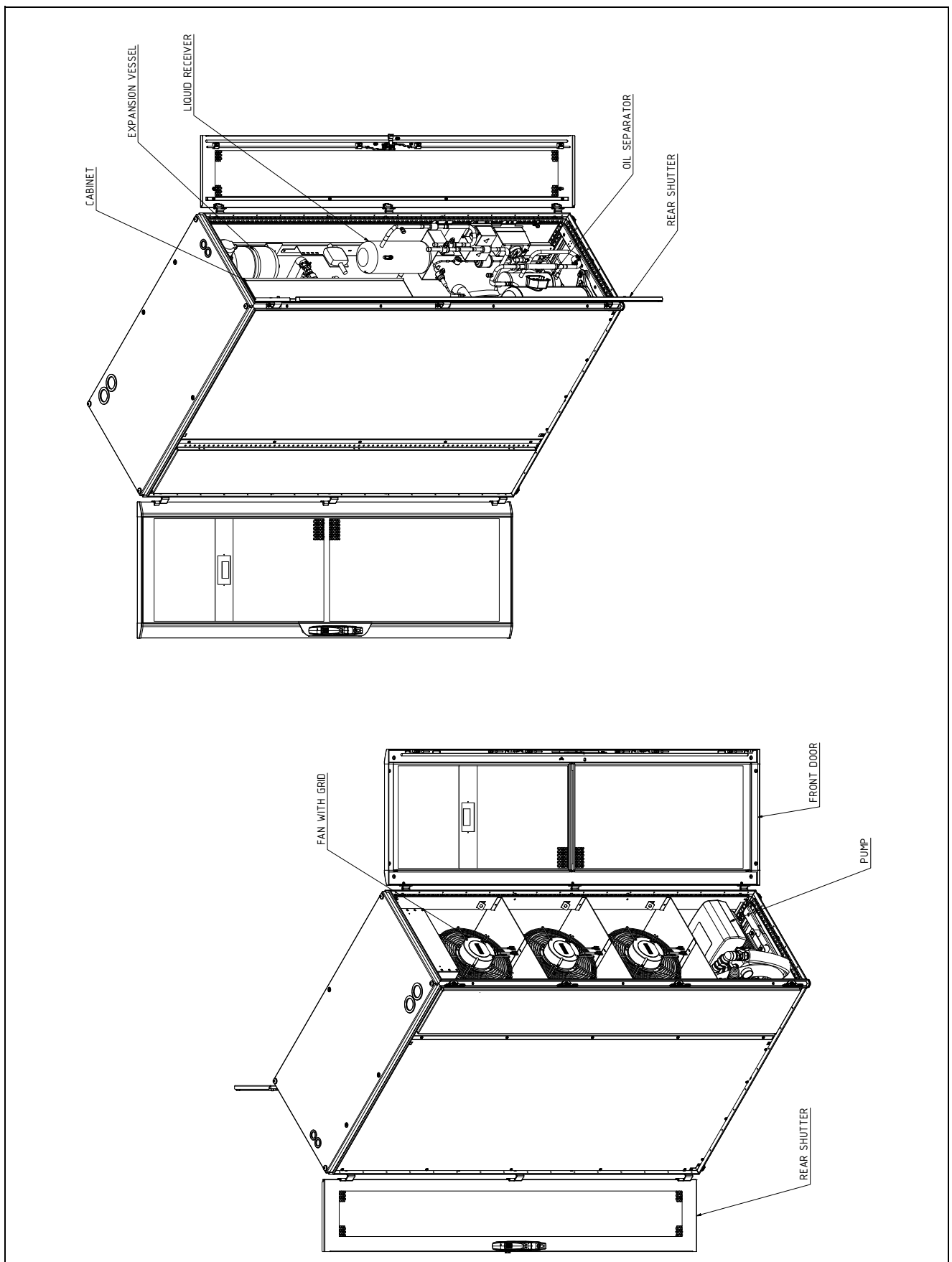
Abb. 72: Übersichtszeichnung 2 LCP DX (1200 mm tief)
