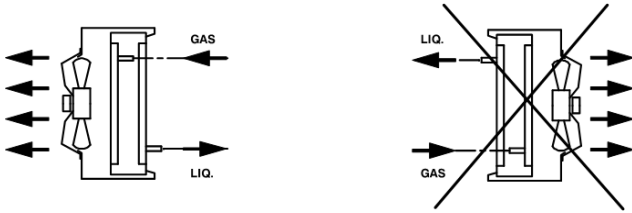
Abb. 17: Verlegung von Heißgas- und Flüssigkeitsleitung
