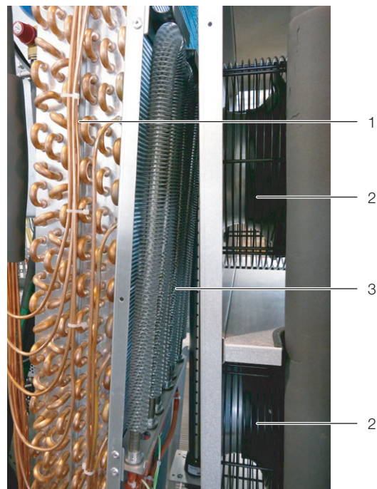
Abb. 56: Elektrische Heizer
