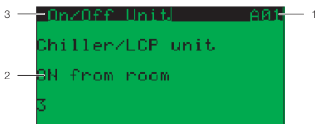
Abb. 34: Menü A01
