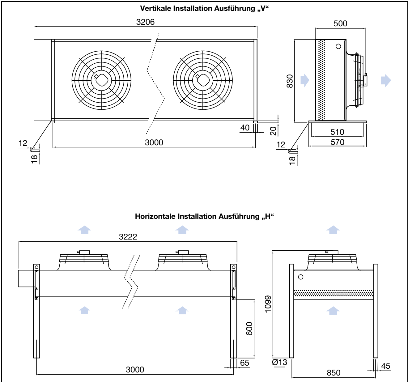
Abb. 75: Aufstellplan des Hochtemperatur-Verflüssigers (3311.XXX)
