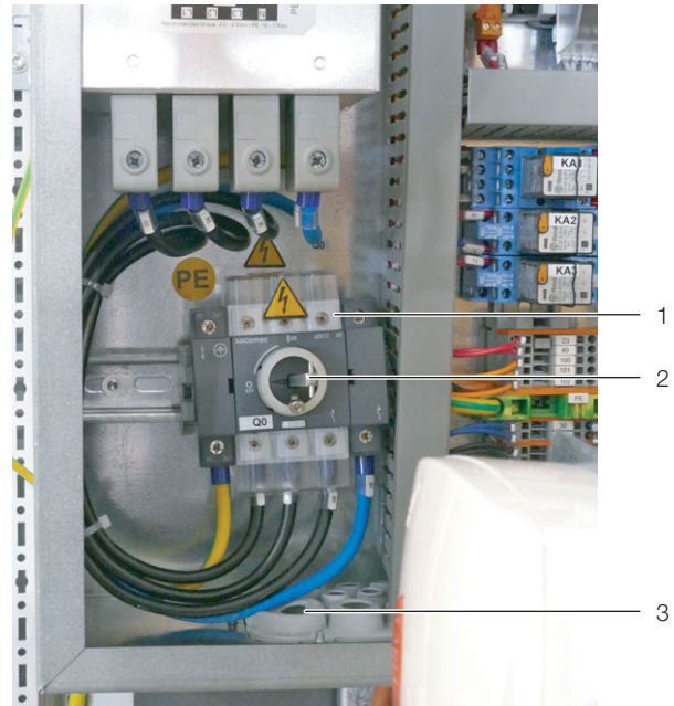
Abb. 25: Geöffnete Elektronikbox
