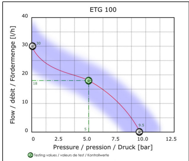
Abb. 63: Leistungsdiagramm der Kondensatpumpe
