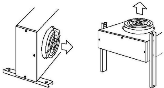
Abb. 16: Horizontale oder vertikale Montage
