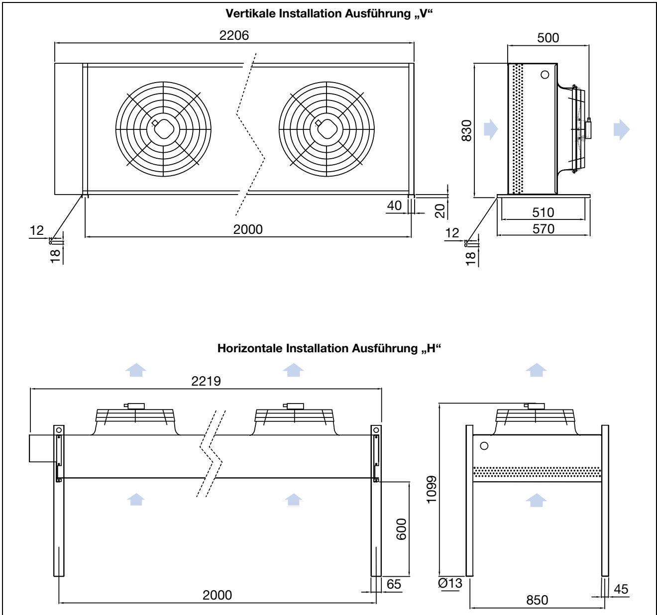
Abb. 73: Aufstellplan des Standard-Verflüssigers 3311.370
