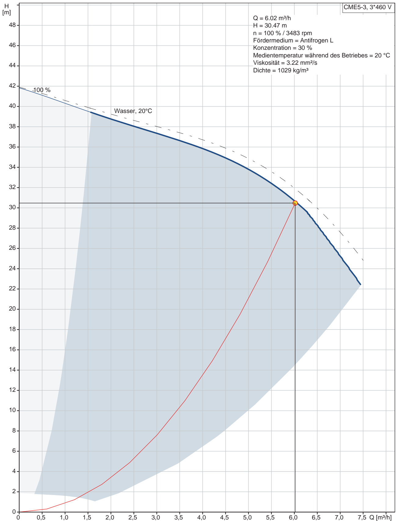
Abb. 84: Kennlinie Kühlwasserpumpe
