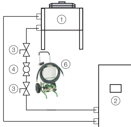
Abb. 22: Zusätzliche Bauteile im Kühlwasserkreislauf
