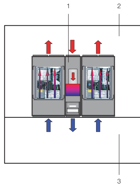
Abb. 10: Aufstellraum mit Kaltgang-Schottung
