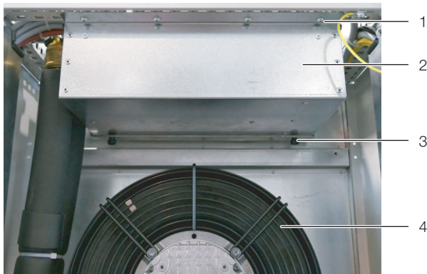
Abb. 59: Zusätzliche Elektronikbox
