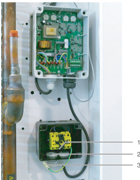
Abb. 27: Elektroanschluss am externen Verflüssiger
