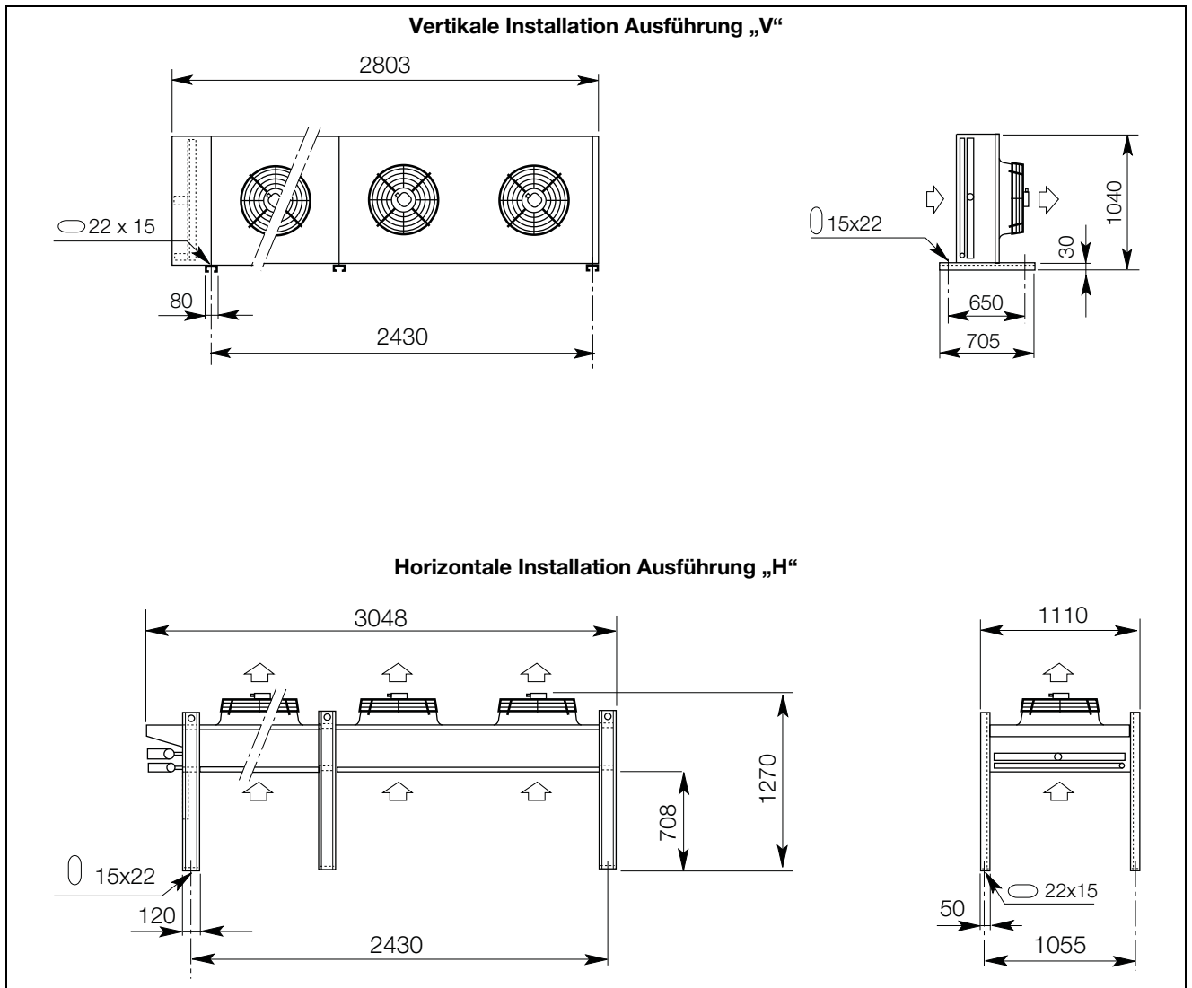
Abb. 74: Aufstellplan des Verflüssigers zur indirekten Freikühlung (3311.380)
