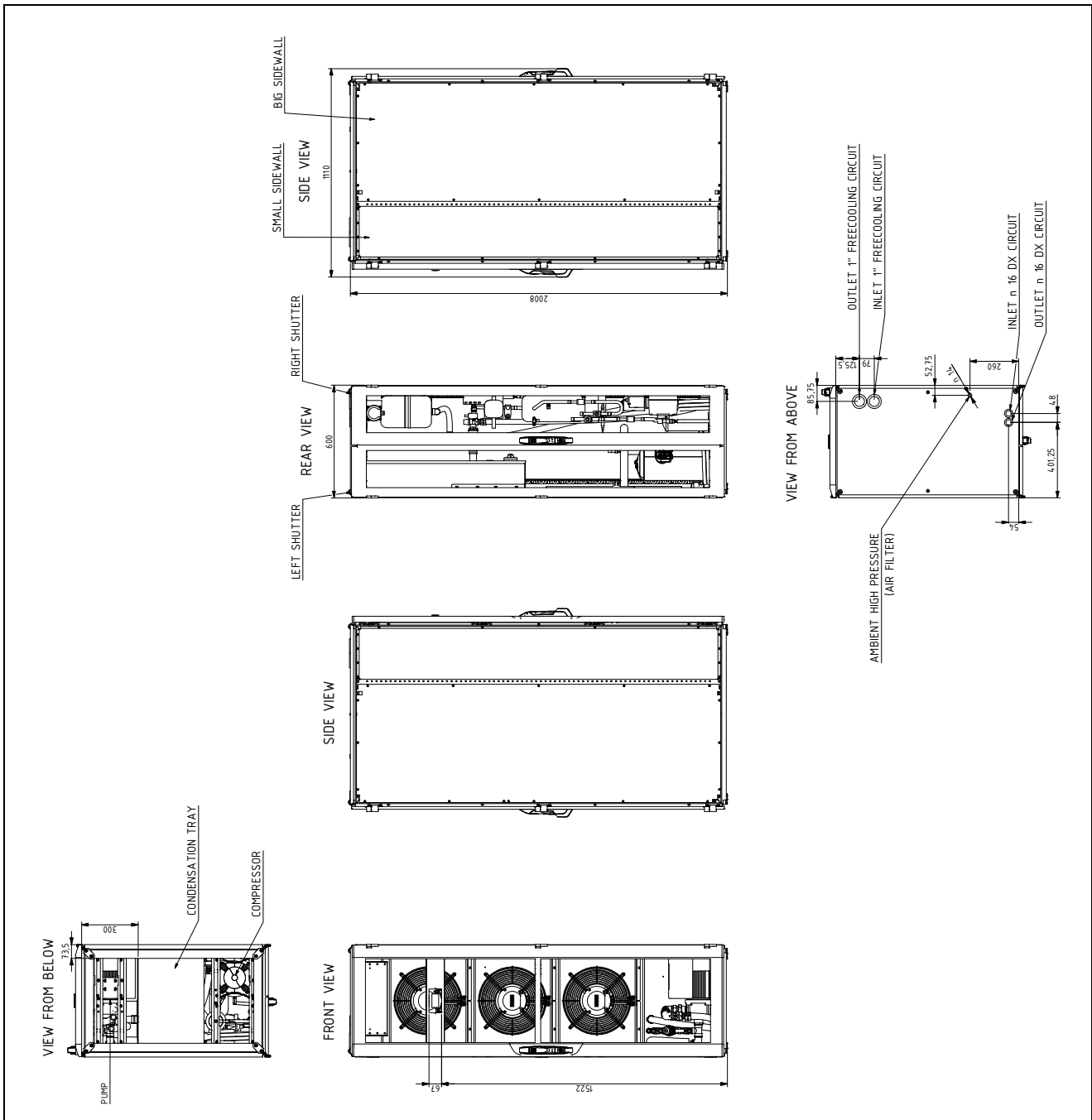
Abb. 69: Übersichtszeichnung 1 LCP DX (1000 mm tief)
