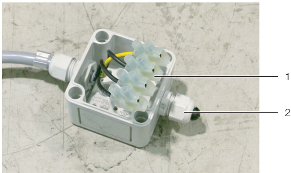
Abb. 30: Elektroanschluss am LCP DX/FC
