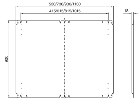
Placa de montagem
