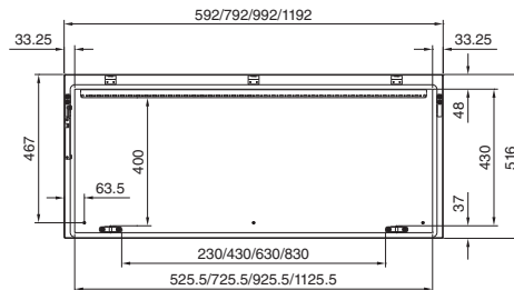
Vista no sentido X
