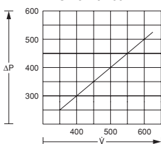
Wasserwiderstandskennlinie SK 3219.100
