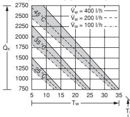
Kennlinienfeld SK 3249.104 (DIN 3168) (50/60 Hz)
