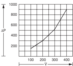
Wasserwiderstandskennlinie SK 3216.100
