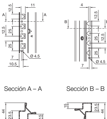
Perfil
