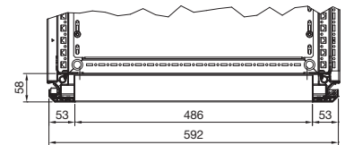
Detalje Y
