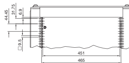
Detail Y
