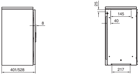
1 parçalı kurulum
