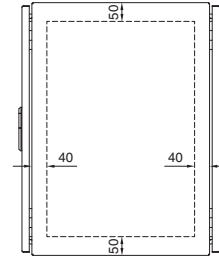
Montaj kesiti
