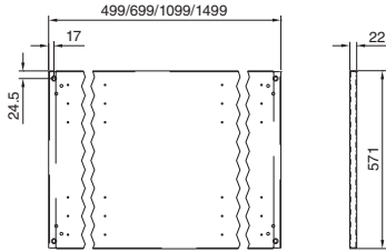
Montaj plakası
