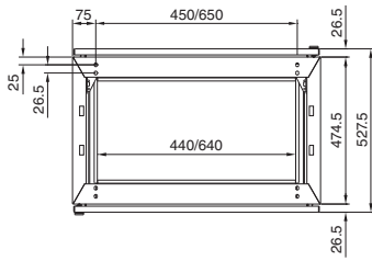
Montaj plakası
