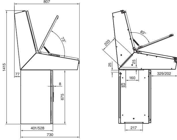
3 parçalı kurulum
