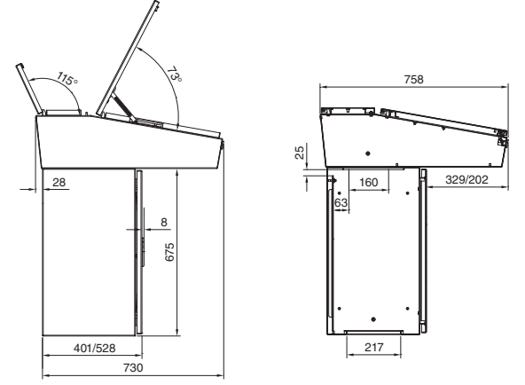
2 parçalı kurulum
