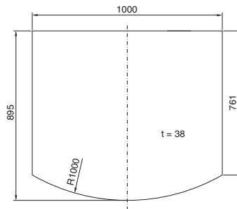
Arbeidsplate IW 6902.100
