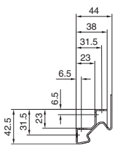
型材横截面
