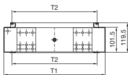
A - A 截面
