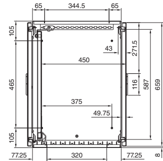
A – A metszet
