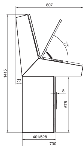
Háromrészes felépítés
