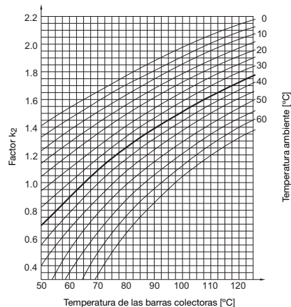
Diagrama del factor corrector según DIN 43 671
