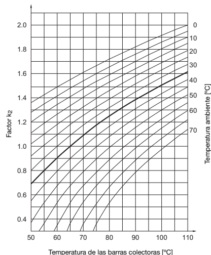
Diagrama del factor corrector para PLS
