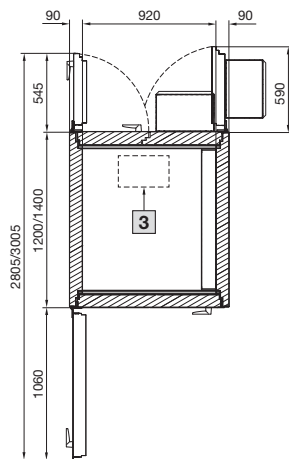
3 Kabelschot in top- of bodemelement als hardschot/bruikbare velden: 2x 120 x 120 mm (optie)
