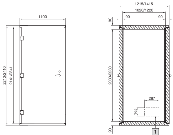
1 Kabelschot als zachtschot (standaard)
