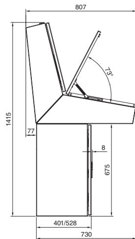
Třídílná sestava
