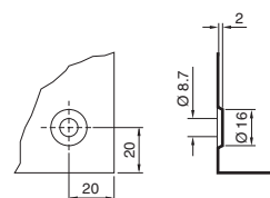
Bemäßung Wandbefestigung
