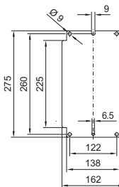
Montageplatte
