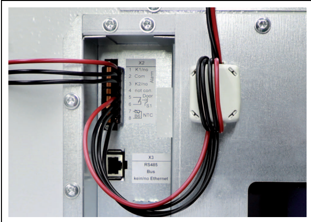
Abb. 32: Montagepunkt des Ferritkerns bei SK 3185330
