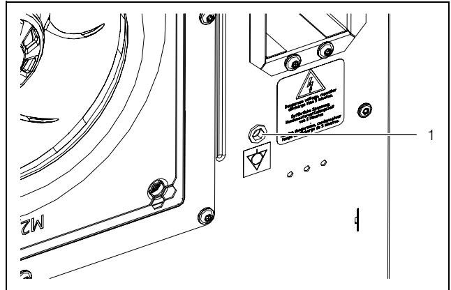
Abb. 34: Anschlusspunkt für Potenzialausgleich (beispielhafte Darstellung)
