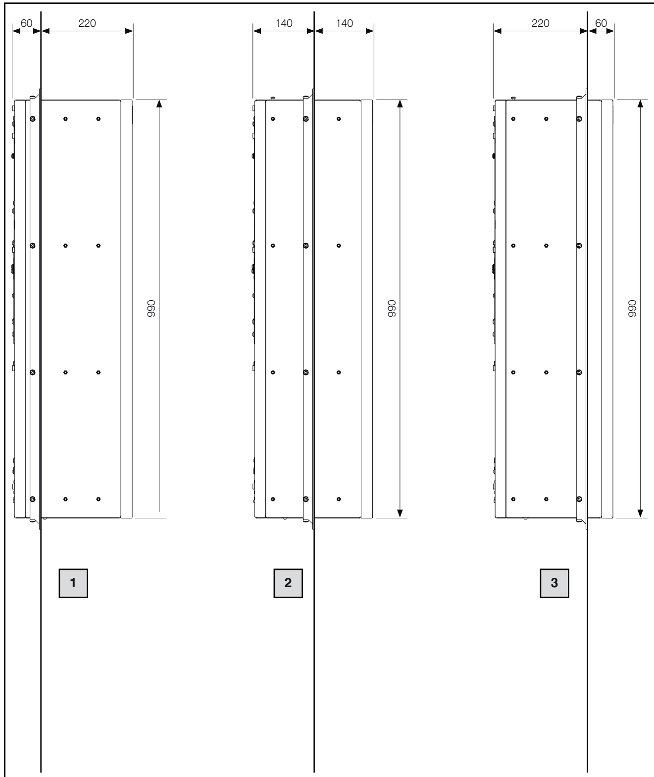
Abb. 53: Abmessungen
