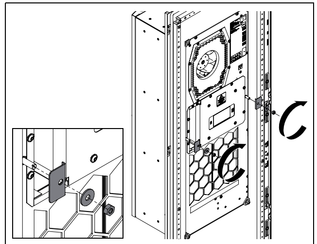
Abb. 18: Montieren der mittleren L-Winkel
