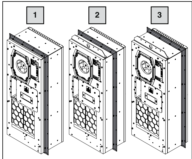
Abb. 20: Mögliche Positionen des Montagerahmens
