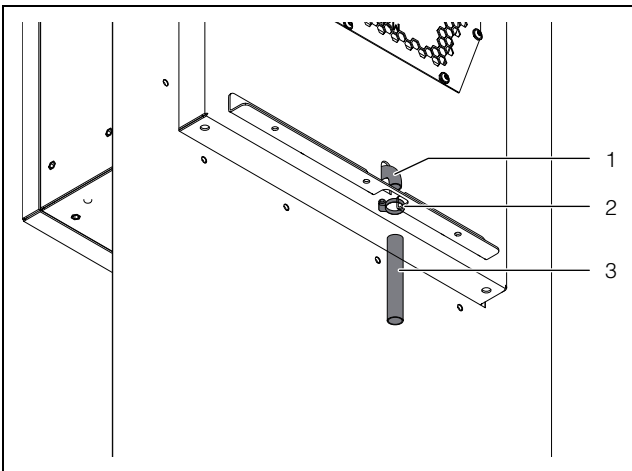
Abb. 30: Anschluss für Kondensatwasserablaufschauch
