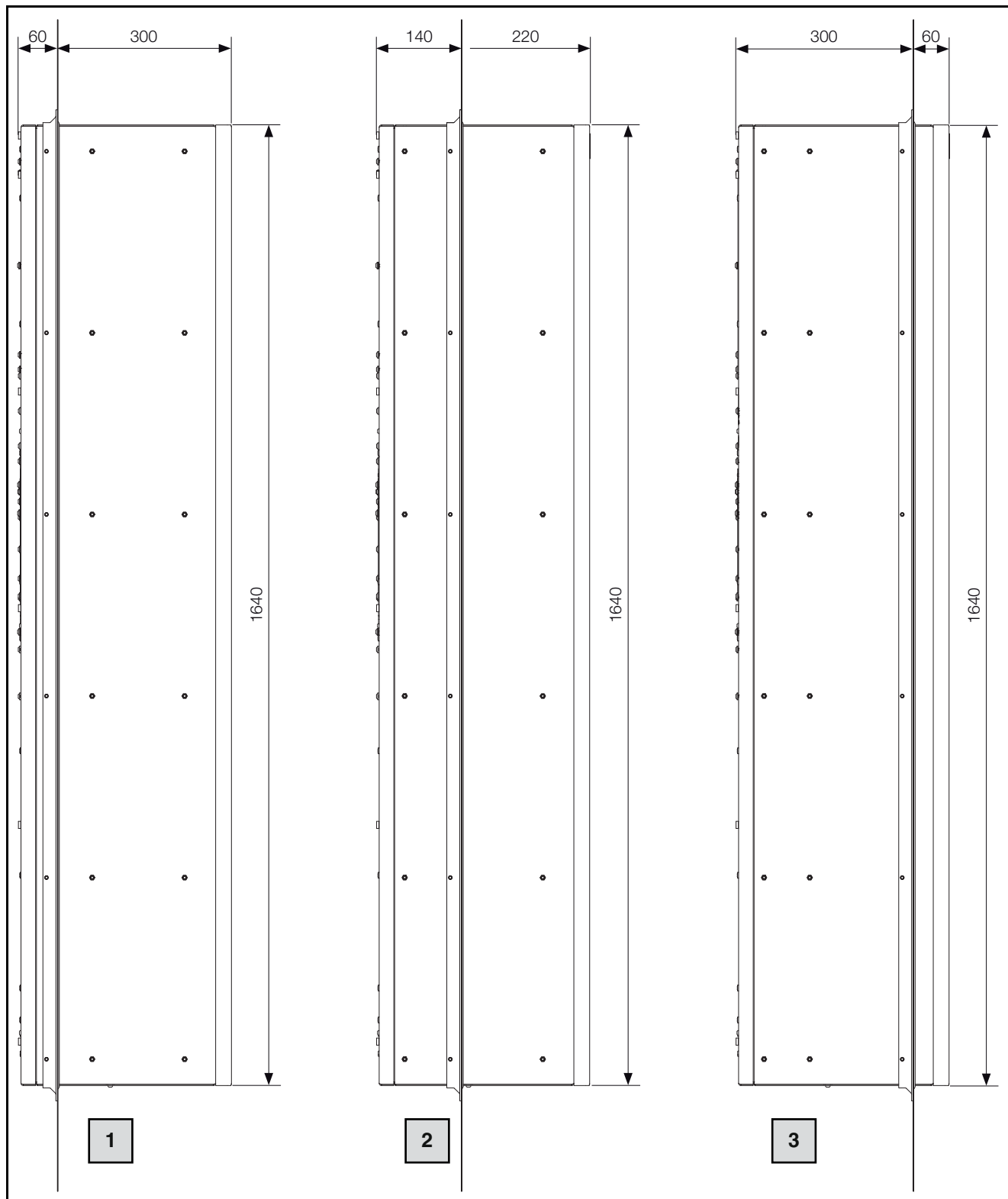
Abb. 55: Abmessungen
