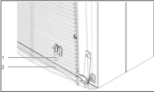
Fig. 12 : raccordement pour le tuyau d'évacuation des eaux de condensation
