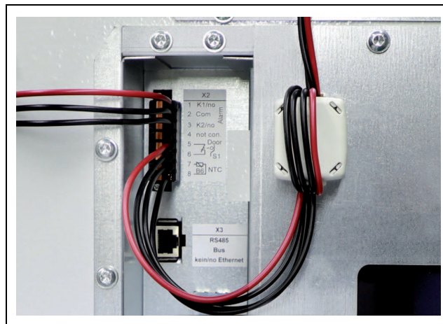
Fig. 14 : câbles de signalisation avec noyau en ferrite monté
