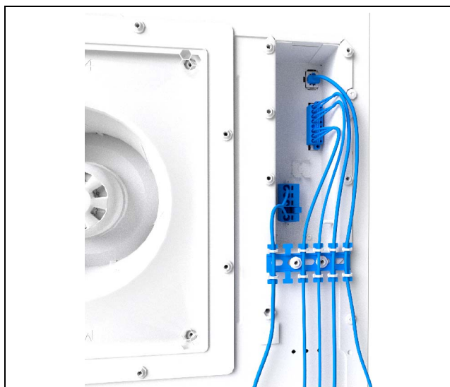
Fig. 20 : réalisation de la décharge de traction à l'aide de colliers de câblage (exemple de représentation)
