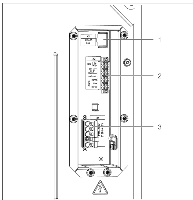
Fig. 13 : ports et connecteurs à l'arrière (exemple de représentation)
