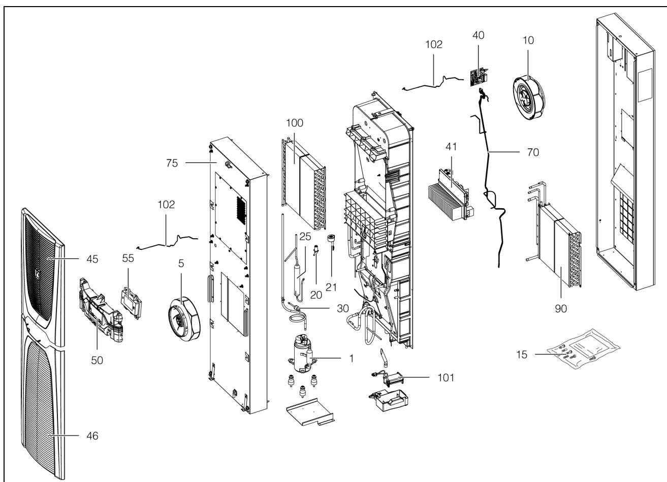
Fig. 37 : pièces de rechange (exemple de représentation)
