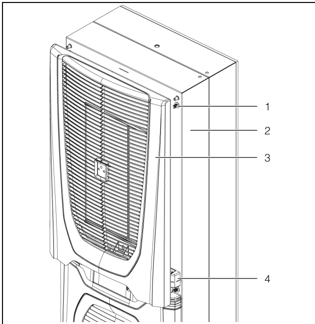
Fig. 29 : ôter la grille à lamelles supérieure (exemple de représentation)
