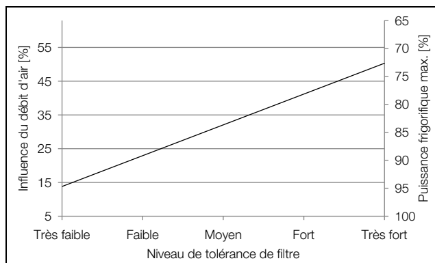
Fig. 25 : exemple de tracé de la puissance frigorifique
