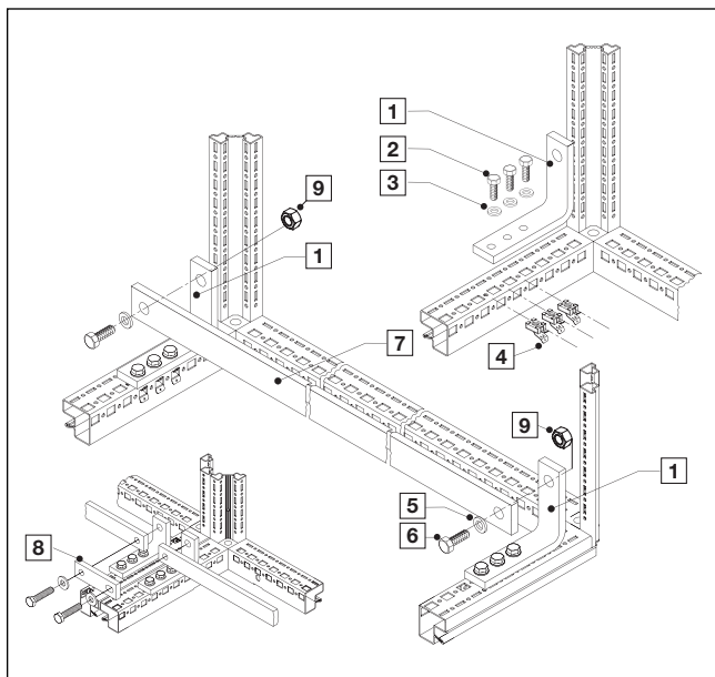
TS 8 – PE/PEN kombinovaný úhelník TS 8 – PE/PEN combination
