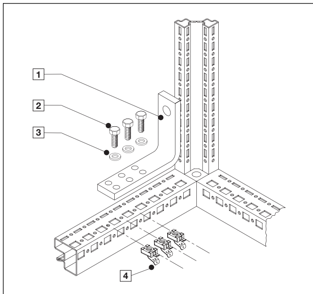
TS 8 – PE/PEN kombinovaný úhelník TS 8 – PE/PEN combination
