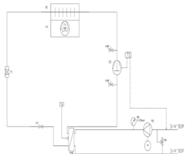
Рис. 2 Контур охлаждения (принципиальная схема, пример: агрегаты с закрытым контуром охлаждающей жидкости)
