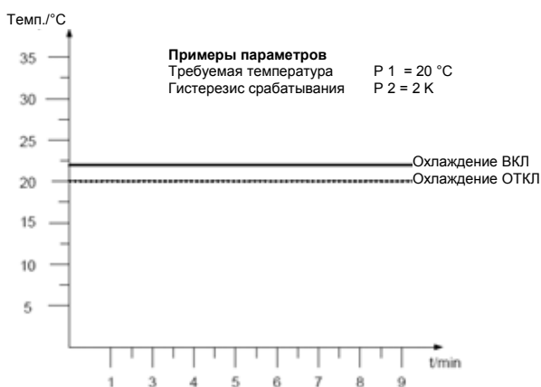
Рис. 5 Регулирование с фиксированным значением, положительный гистерезис
