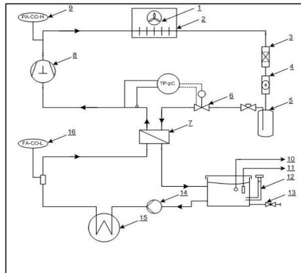
Рис. 1 Контур охлаждения (пример: агрегаты с открытым контуром охлаждающей жидкости)
