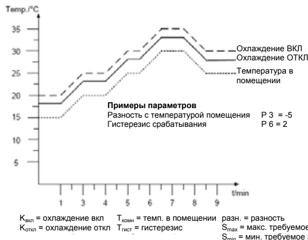
Рис. 6 Регулирование в зависимости от температуры помещения
